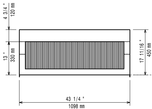
Zij aanzicht
